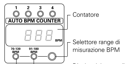
Display BPM
